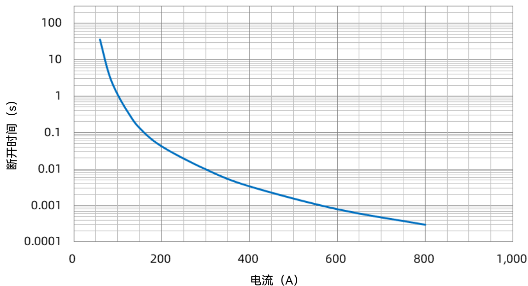
SHP 30 A 电流-时间曲线
