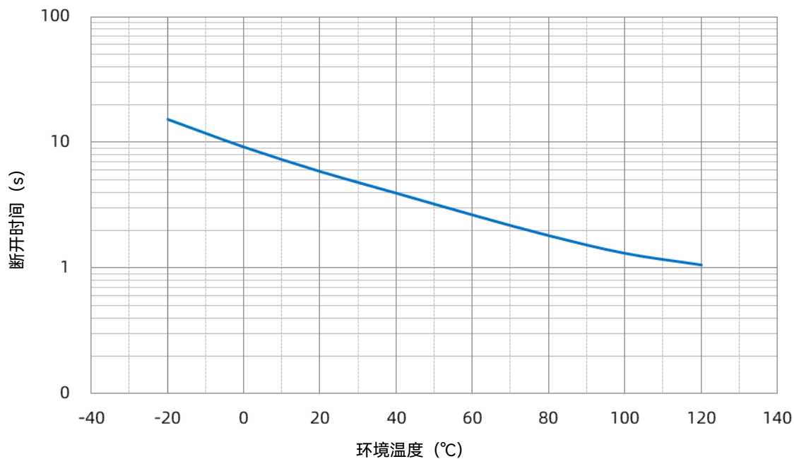
SHP 75 A 温度-时间曲线
