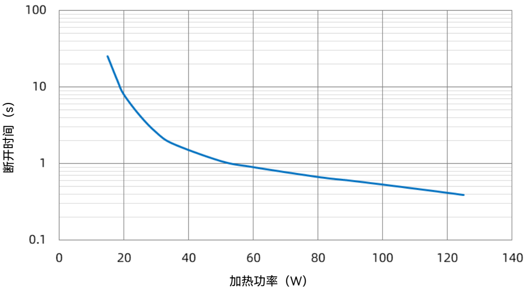
SHP 45 A 功率-时间曲线
