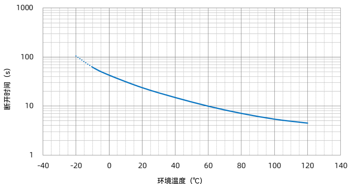
SHP 30 A 温度-时间曲线
