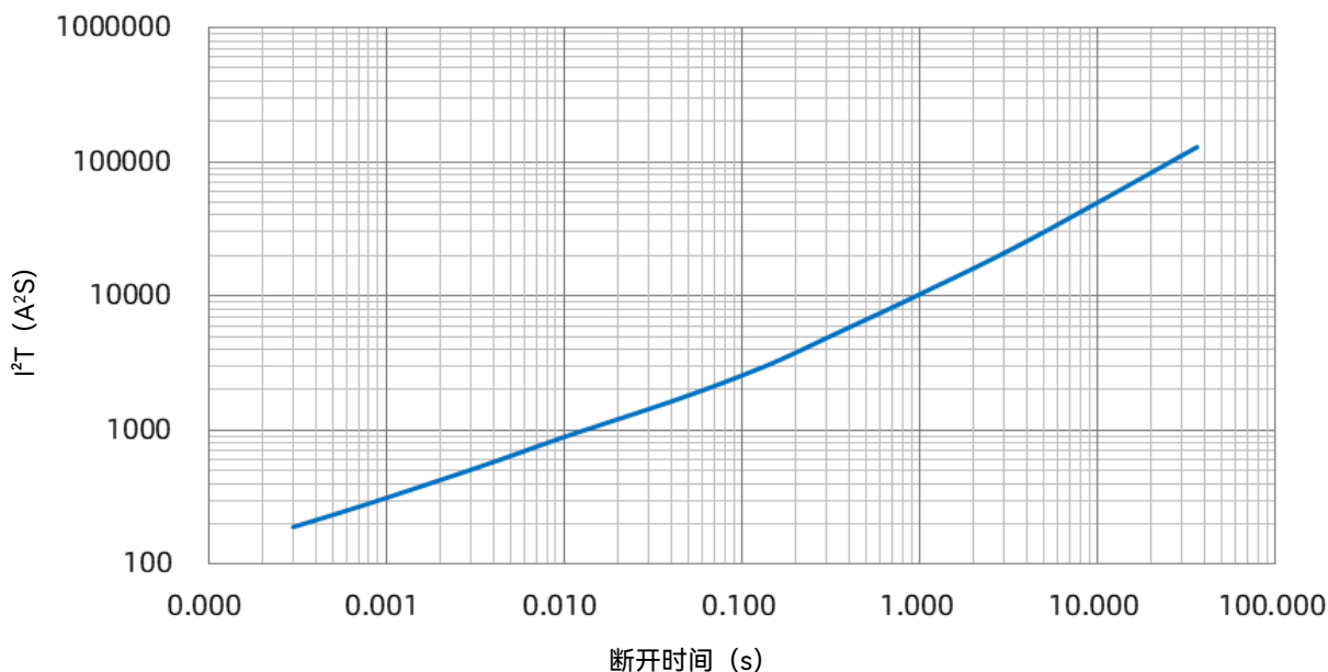
SHP 30 A I 2 t-t 曲线
