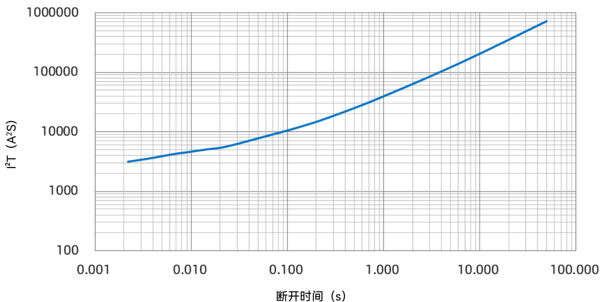
SHP 75 A I 2 t-t 曲线
