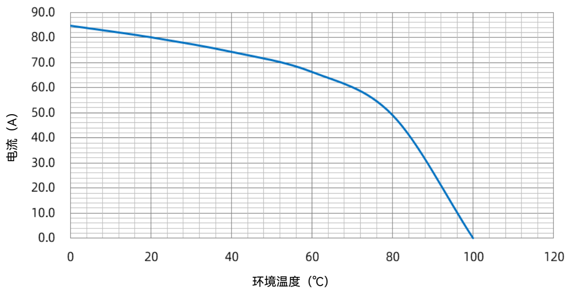
SHP 75 A 载流能力曲线
