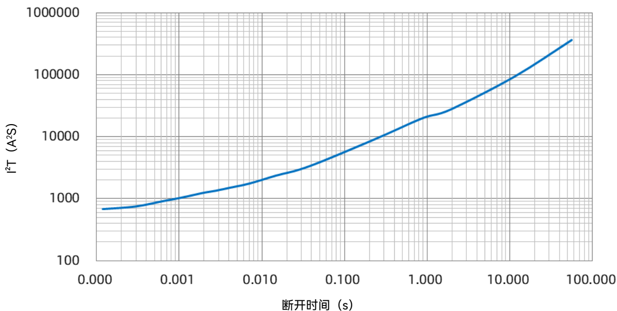
SHP 45 A I 2 t-t 曲线
