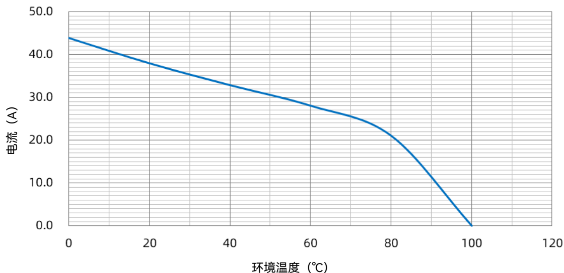
SHP 30 A 载流能力曲线
