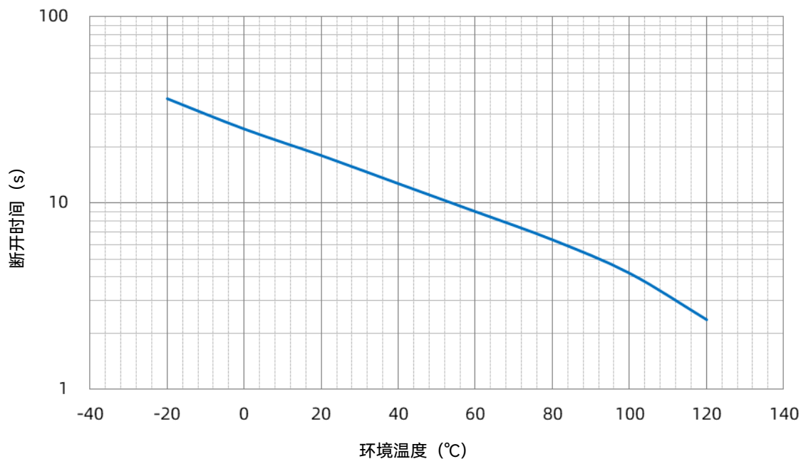
SHP 60 A 温度-时间曲线
