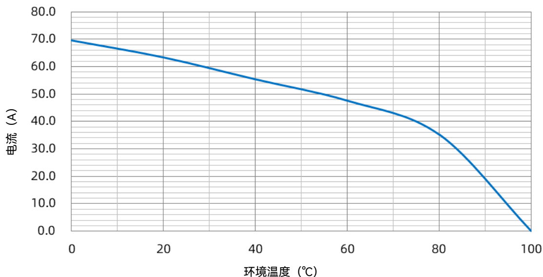
SHP 60 A 载流能力曲线
