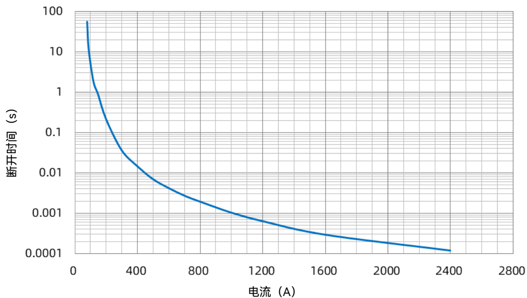
SHP 45 A 电流-时间曲线
