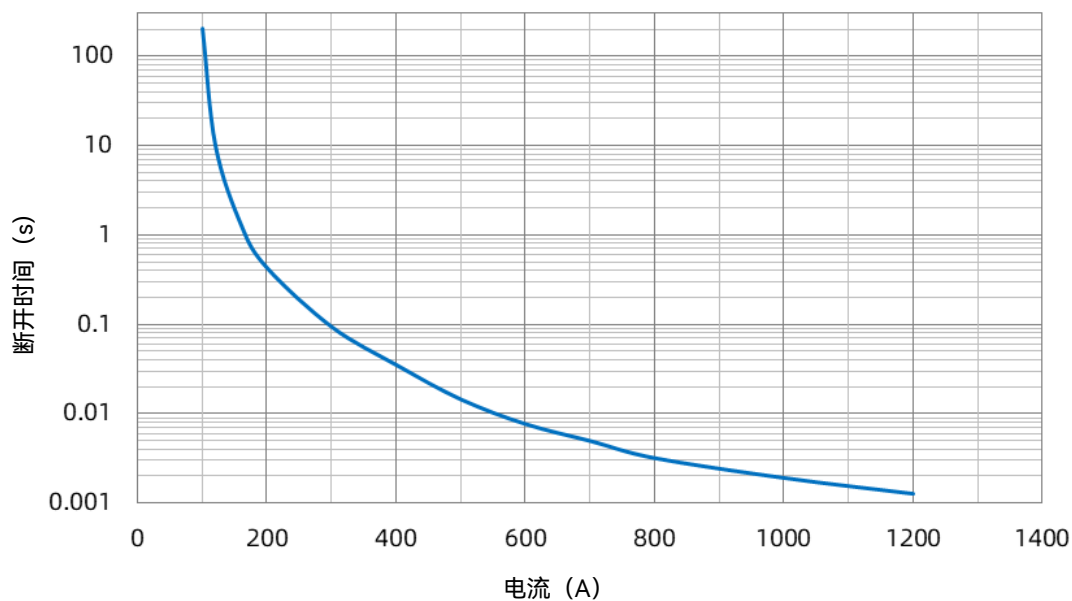
SHP 60 A 电流-时间曲线
