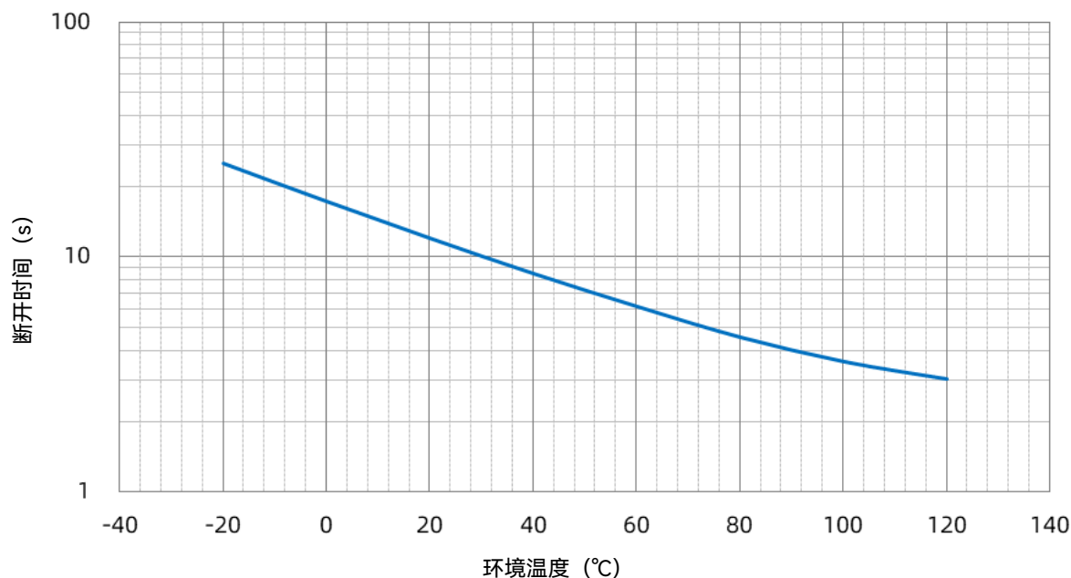
SHP 45 A 温度-时间曲线
