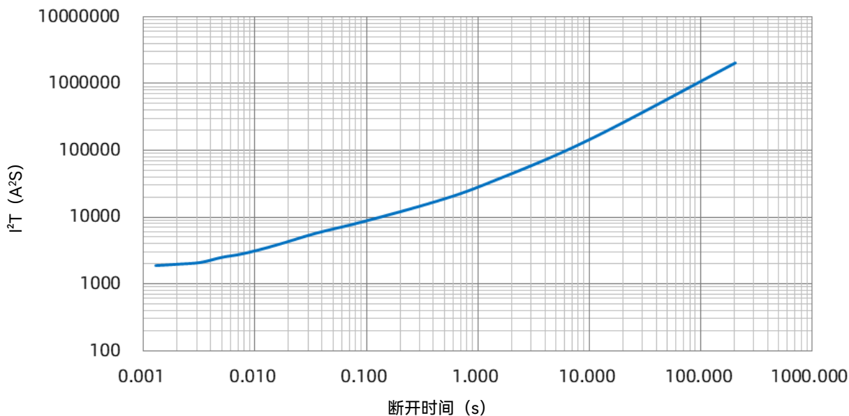
SHP 60 A I 2 t-t 曲线
