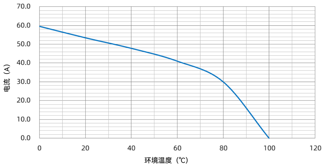
SHP 45 A 载流能力曲线
