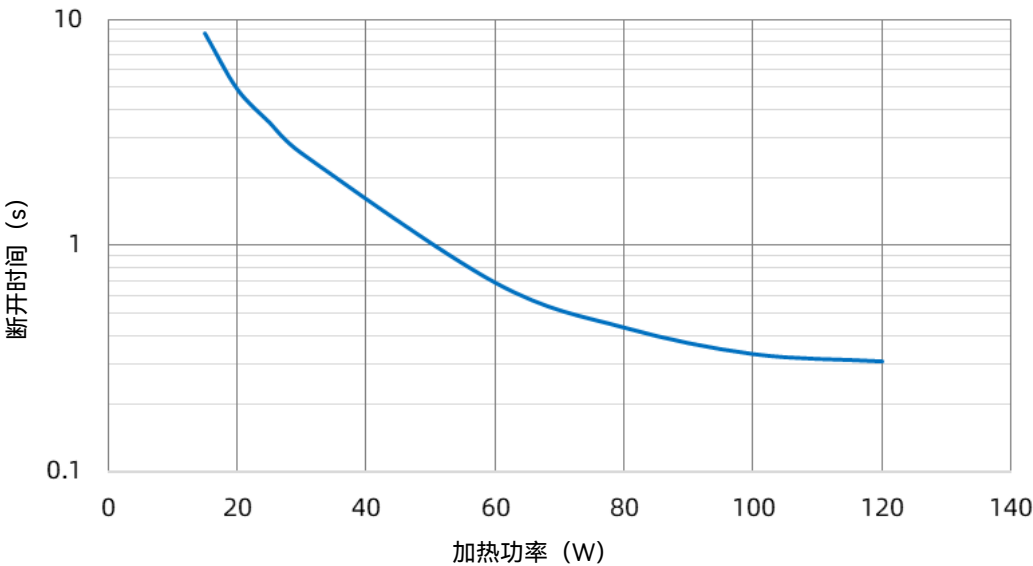
SHP 30 A 功率-时间曲线
